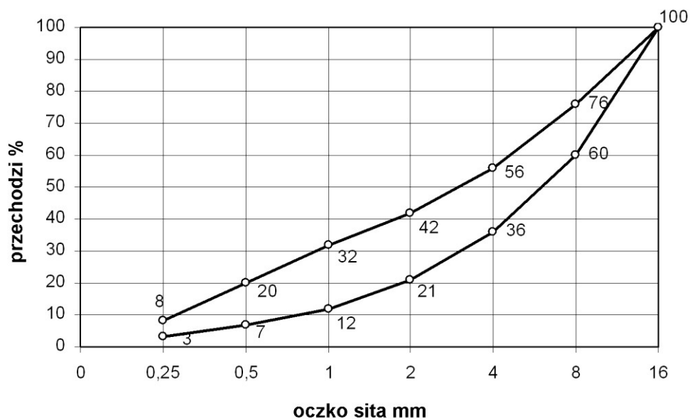
Rysunek 1. Graniczne krzywe uziarnienia kruszywa 0 \square 16 mm (dla betonu klasy C25/30)
