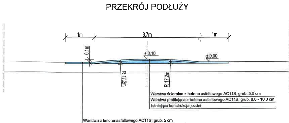
Rys. 1 Przekrój podłużny liniowego progów zwalniających
