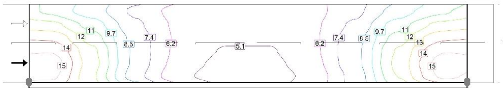
Wartości konserwacji, poziome natężenie oświetlenia [lx] (Izoluxy)
