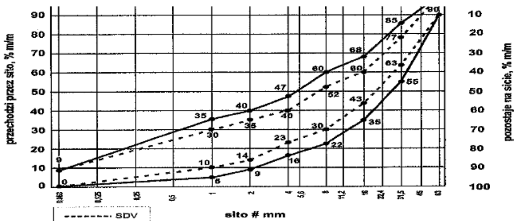
Rys. 14. Mieszanka niezwiązana 0/63 do warstw podbudowy zasadniczej
