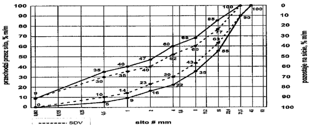
Rys. 12. Mieszanka niezwiązana 0/31, 5 do warstw podbudowy zasadniczej
