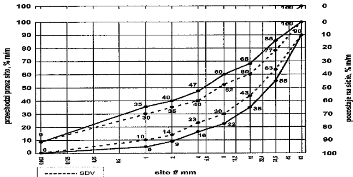
Rys. 14. Mieszanka niezwiązana 0/63 do warstw podbudowy zasadniczej
