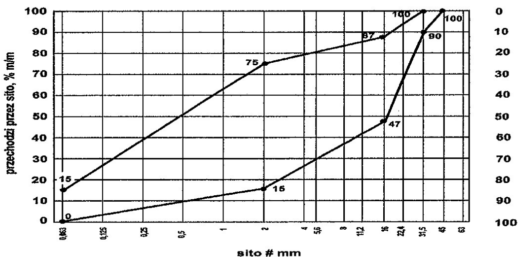
Rys.1. Mieszanka niezwiązana 0/31,5 do podbudowy i nawierzchni z kruszywa
