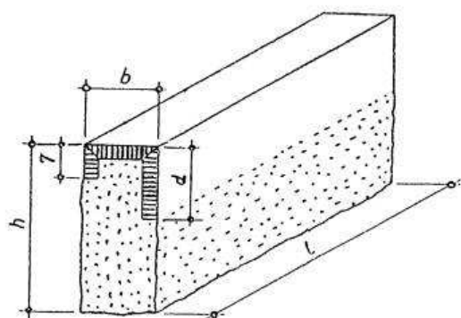
Tablica 2. Wymiary krawężników ulicznych
