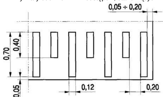
Rys. 2. Oznakowanie poziome progu zwalniającego
