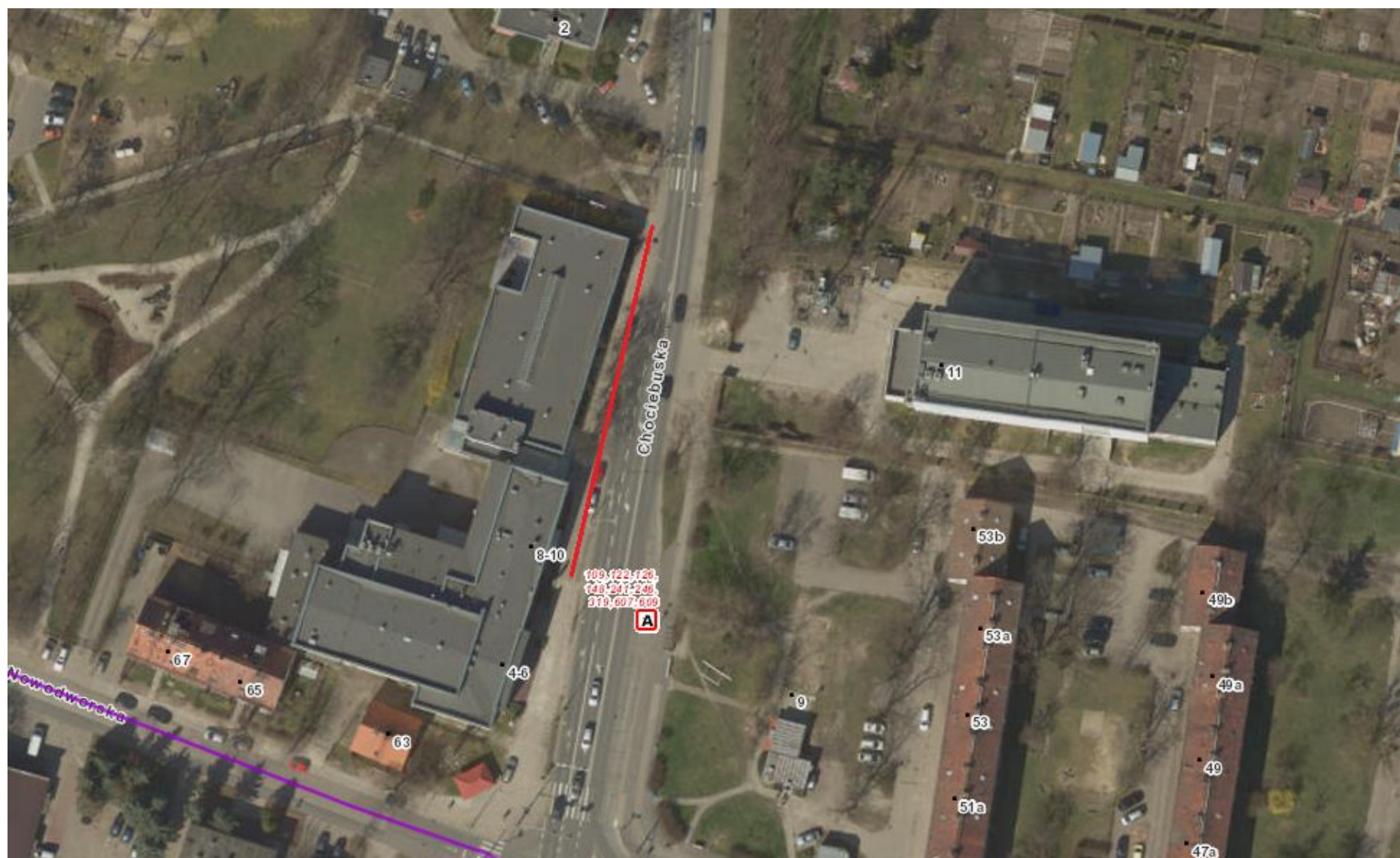
Ul. Chociebuska – mapa poglądowa z planowanym zakresem robót
