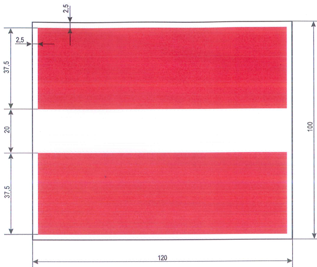
Rys. – znak A.1. - zakaz przejęcia
