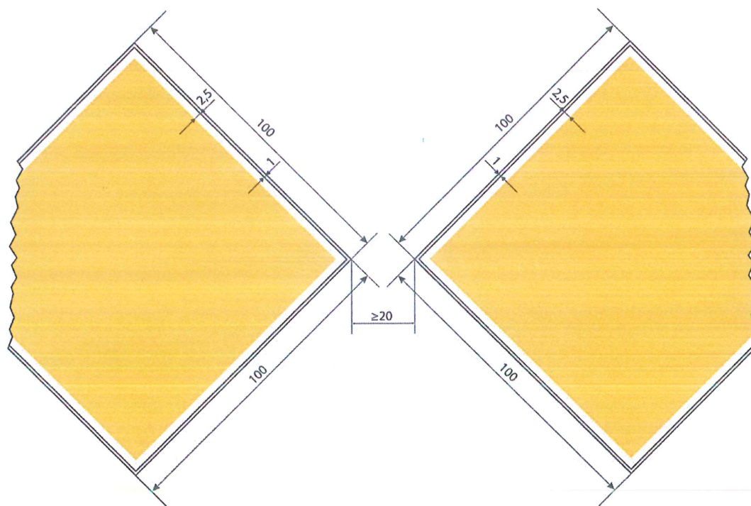
Rys. – znak D.1b – zalecenie przejścia w jednym kierunku (przejście z przeciwnego kierunku zabronione)
