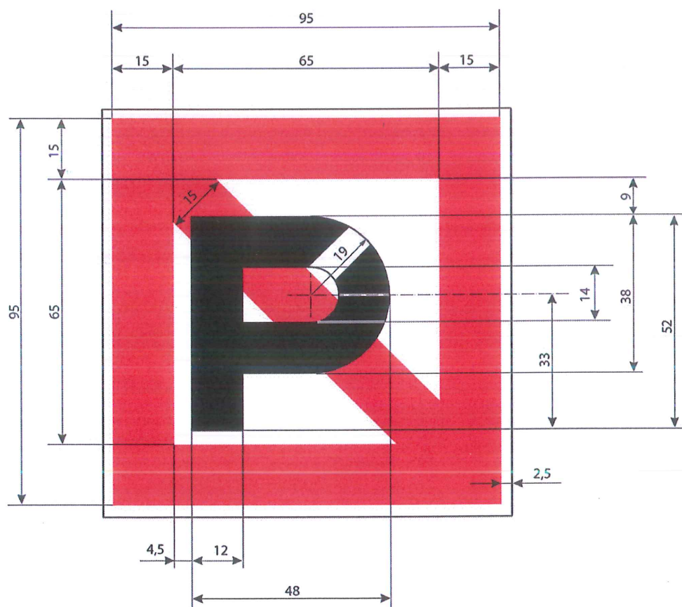
Rys. – znak A.5 - zakaz postoju (na kotwicy lub na cumach przy brzegu)
