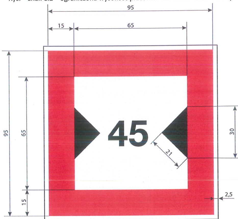
Rys. – znak C.3 – Ograniczona szerokość szlaku lub kanału żeglownego
