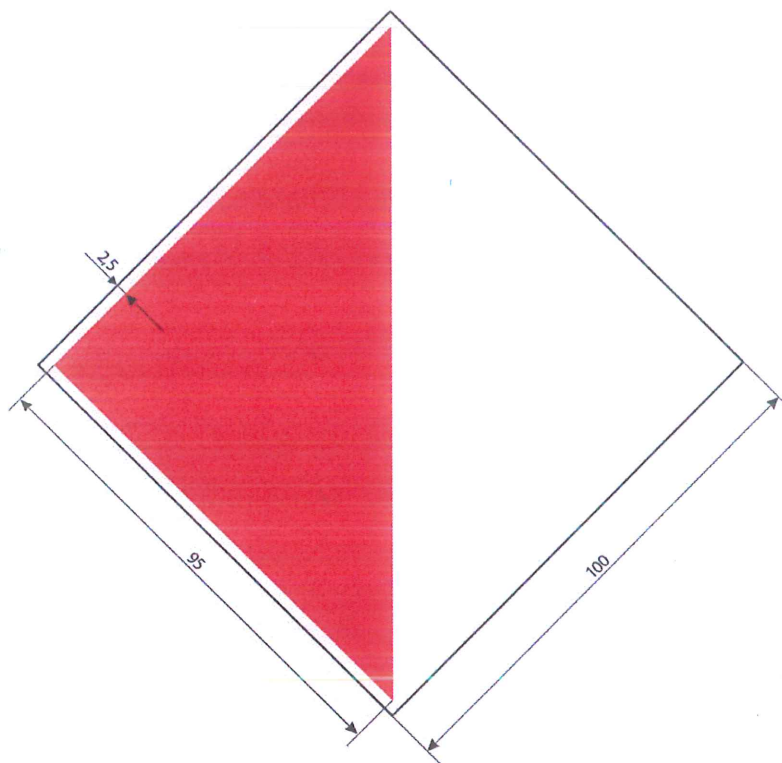
Rys. – znak A.10 – zakaz przejścia poza skrajnią określoną tablicami (pod mostem)
