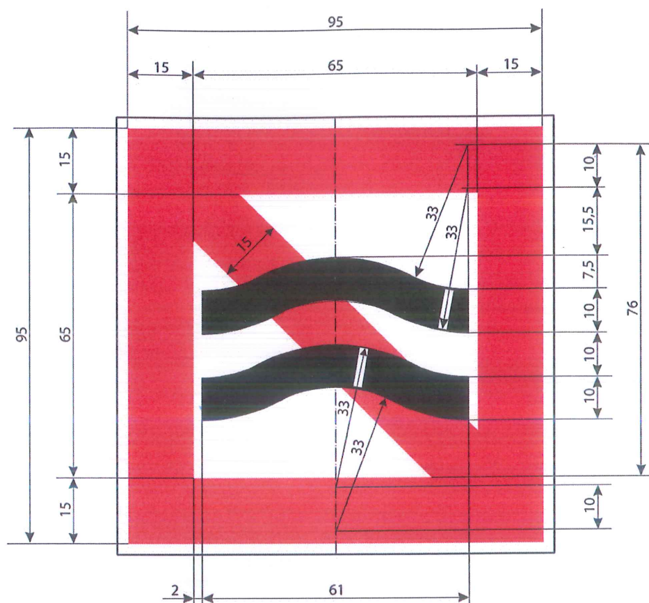
Rys. – znak A.9 – zakaz wytwarzania fali
