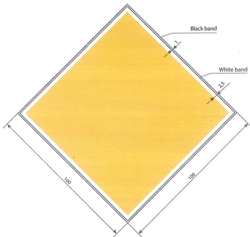
Rys. – znak D.1a – zalecenie przejścia w obydwu kierunkach
