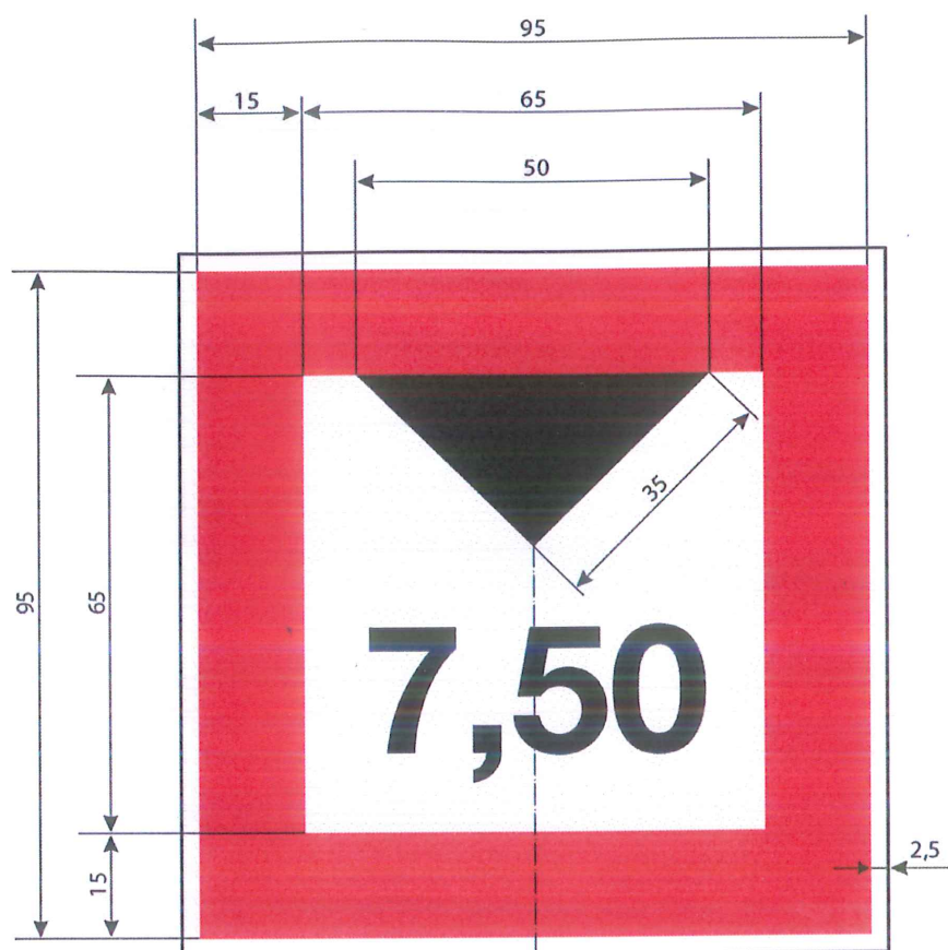
Rys. – znak C.2 – ograniczona wysokość prześwitu nad zwierciadłem wody
