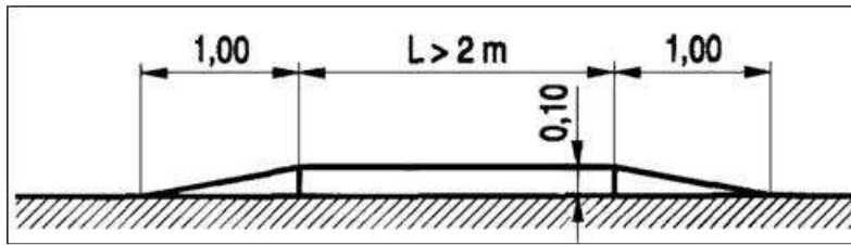
Rys. 4. Przekrój podłużny liniowego proggu zwalniającego listwowego o ograniczonej prędkości przejazdu 18 ÷ 20 km/h (U-16d)
