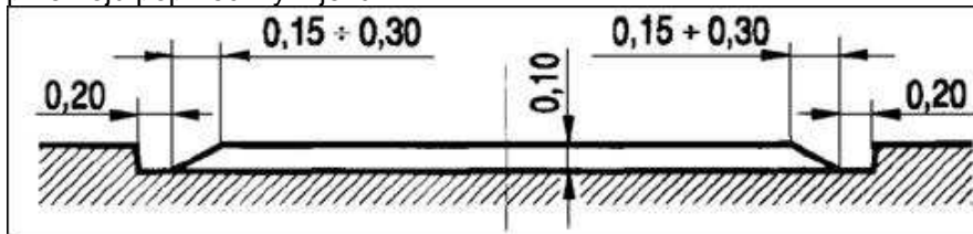
Rys. 5. Przekrój poprzeczny proggu zwalniającego liniowego o zmniejszonej szerokości (proggu skróconego) w przekroju poprzecznym jezdni
