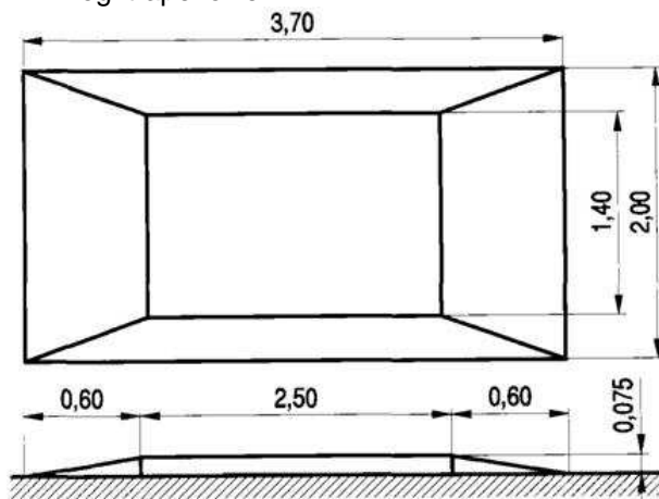
Rys. 2. Przykłady wymiarowania progów zwalniających wyspowych (wg [23]) 2.1. Progi trapezowe
