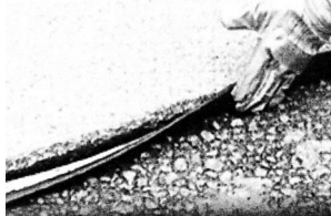
Rys. 2. Docisnięcie taśmy topliwiej dłonią w rękawicy poprzez papier przekładkowy, stroną z klejem zwróconą do powierzchni uszczelnianej
