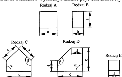
.Rysunek 1. Rodzaje płyt chodnikowych betonowych
