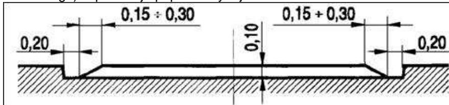
Rys. 5. Przekrój poprzeczny progów zwalniającego liniowego o zmniejszonej szerokości (progów skróconego) w przekroju poprzecznym jezdni
