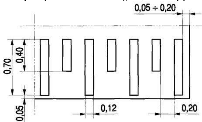
Rys. 2. Oznakowanie poziome progów zwalniających
