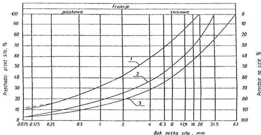
Rysunek 1. Pole dobrego uziarnienia kruszyw przeznaczonych na podbudowy wykonywane metodą stabilizacji mechanicznej 1-2 kruszywo na podbudowę zasadniczą (górną warstwę) lub podbudowę jednowarstwową 1-3 kruszywo na podbudowę pomocniczą (dolną warstwę)
