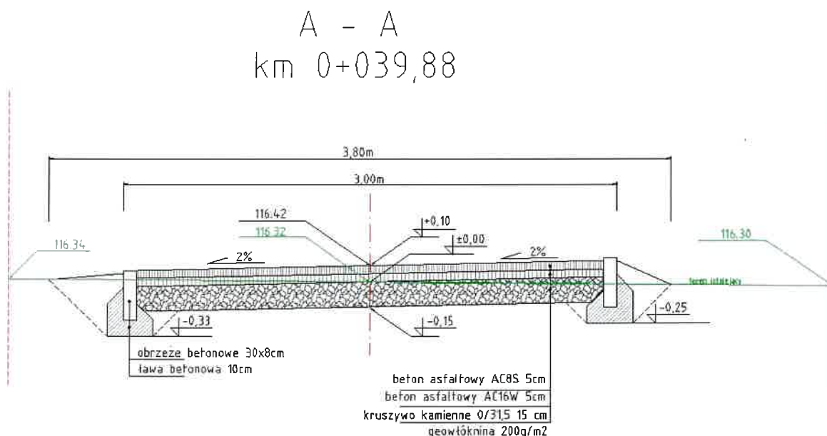
Rys. 1 Przekrój przyjętej konstrukcji
